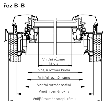
řez B-B
