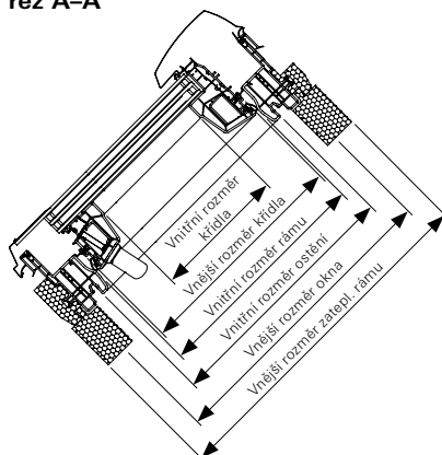
řez A-A
