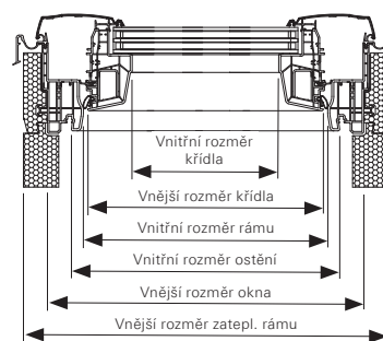
řez B-B
